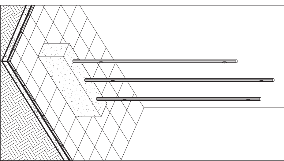
PERSPECTIVA AXONOMETRICA S/ ESCALA
