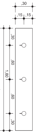
VISTA SUPERIOR
