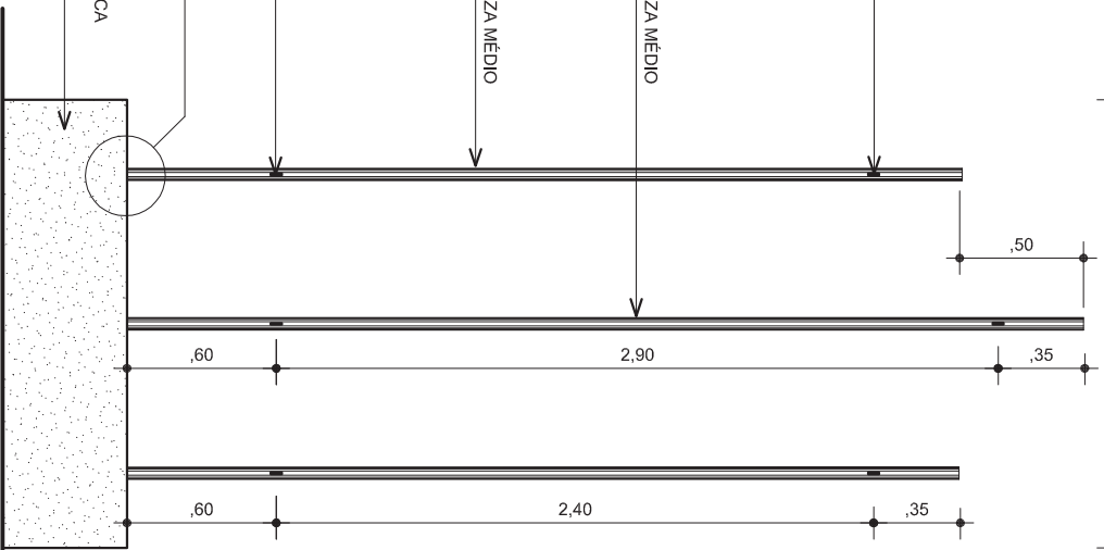
VISTA LATERAL
